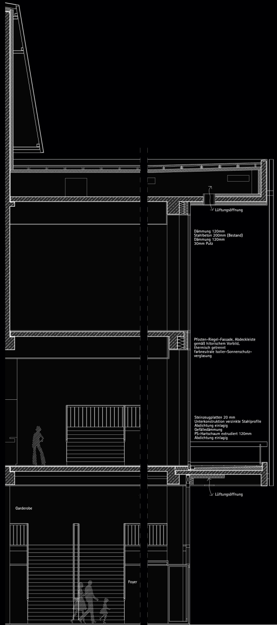
Fassadenschnitt M. 1:50
